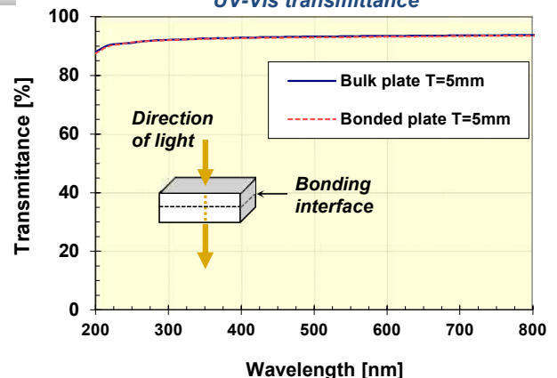
紫外可視分光透過率 UV-Vis transmittance
